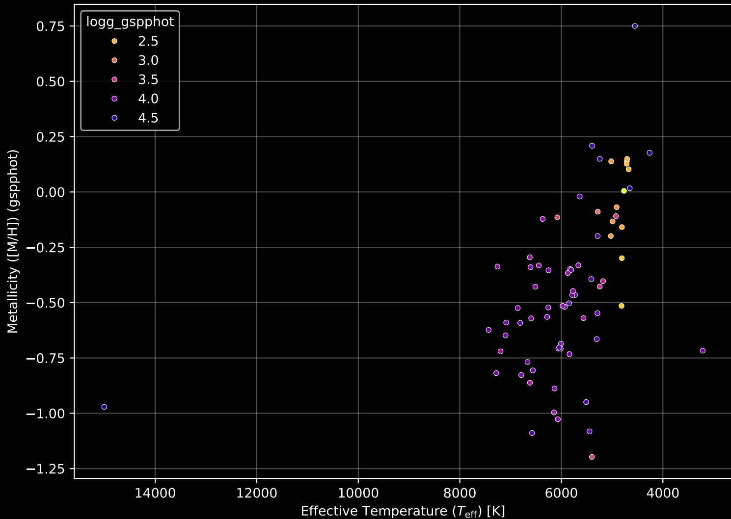
GALAH DR4 Field: [6791] Stellar Population Parameters (n= 73)
